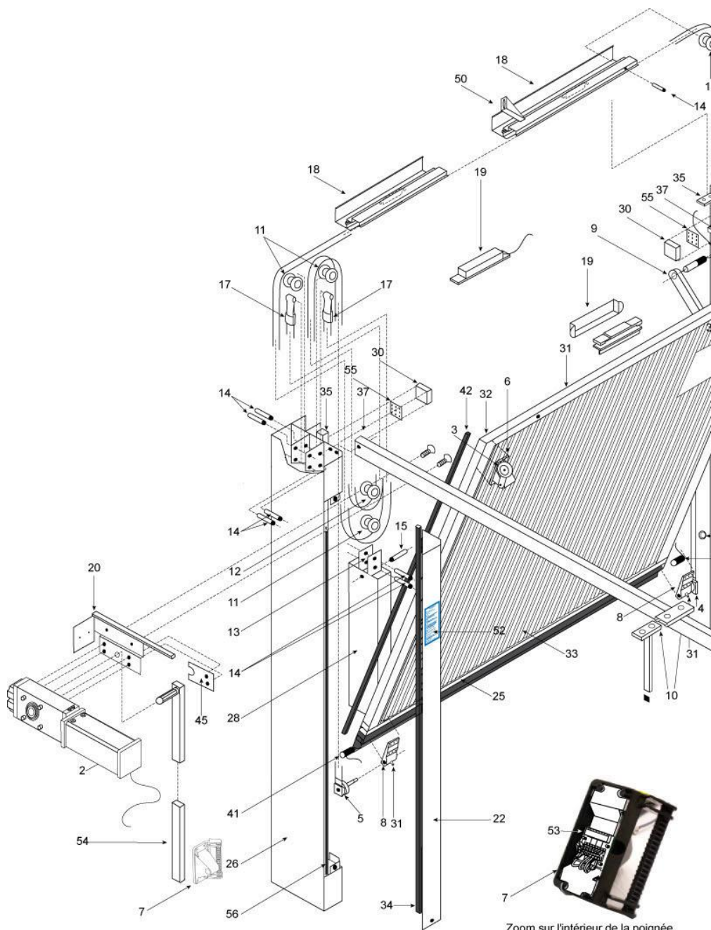
Zoom sur l'intérieur de la poignée
